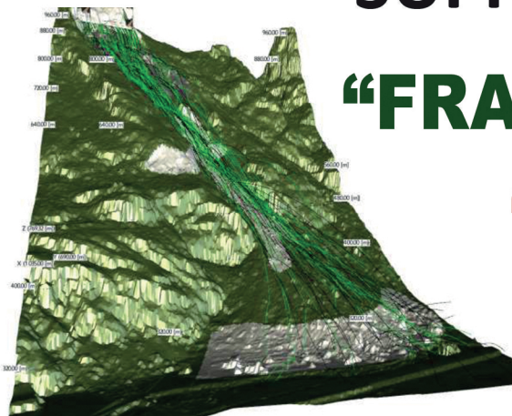
- Simulazione caduta massi in località Chiappetti -
